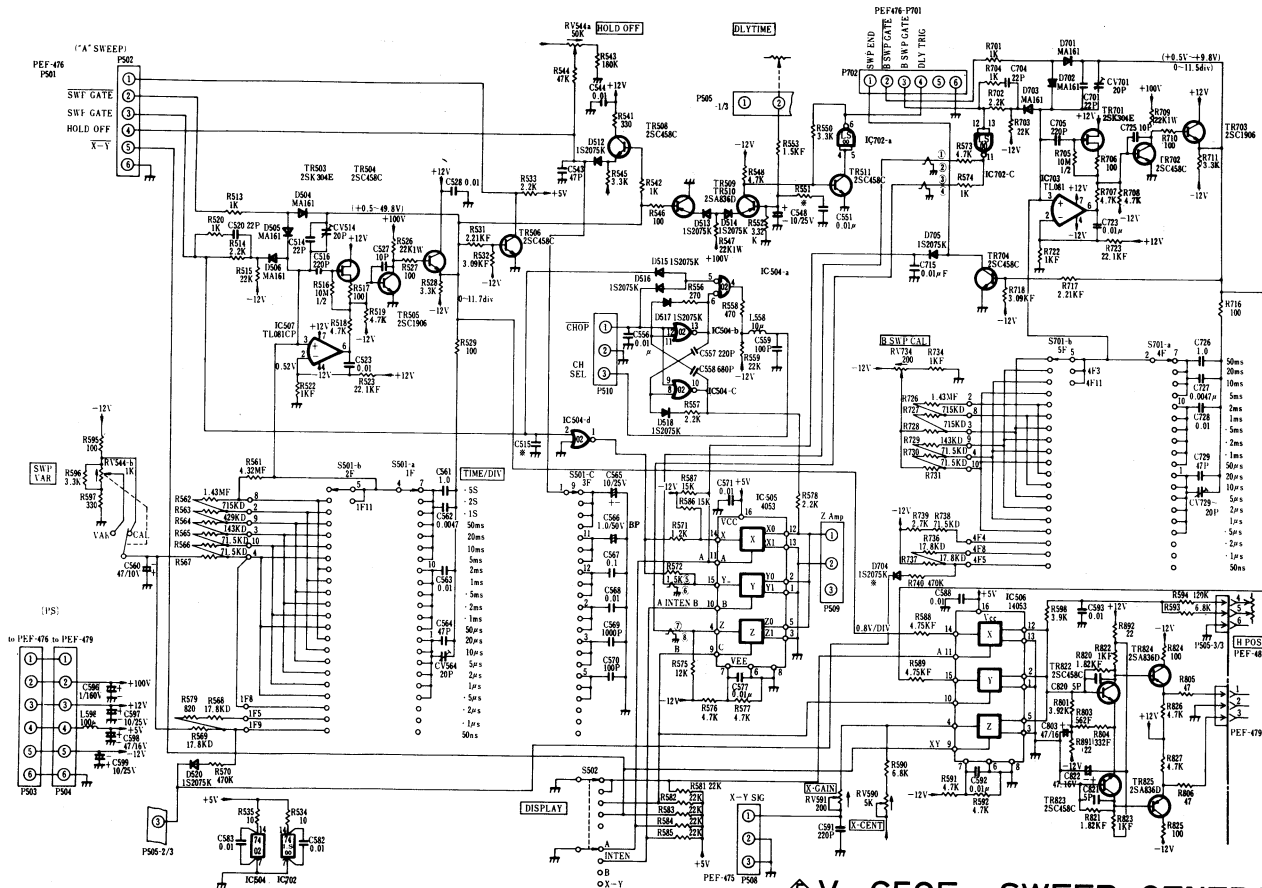
◆ V-650F SWEEP GENERATOR
